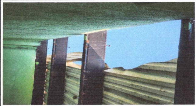
Foto 2: en esta fotografía se observa el deterioro el soporte del metal y la cubierta de lámina.
