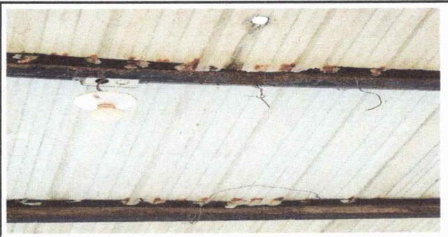
Foto 6: en esta fotografía se observa la estructura de soporte en mal estado y la cubierta de lámina agujereada.
