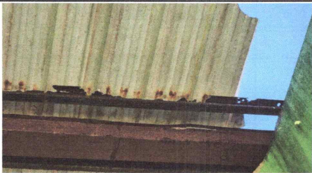
Foto 3: en esta fotografía se observa que la estructura del soporte, esta en mal estado.
